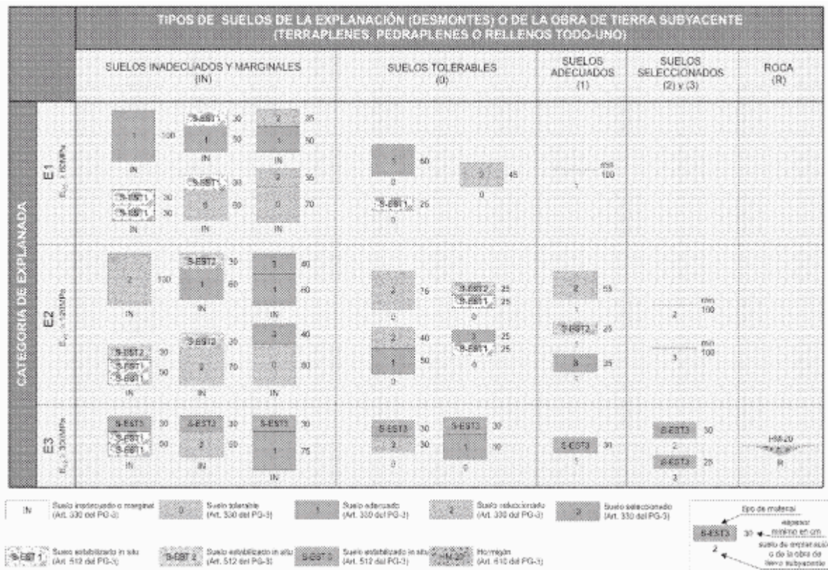
2.1.1.10 FIGURA 1. FORMACIÓN DE LA EXPLANADA.
